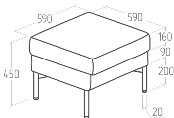
EV-GM-PF.01 590x590x450
