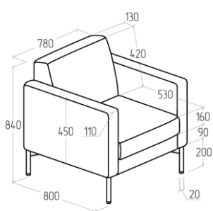
EV-GM-P.01 780x800x840
